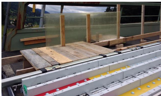
Neue Anlaufspur HS89 mit doppeltem Boden
